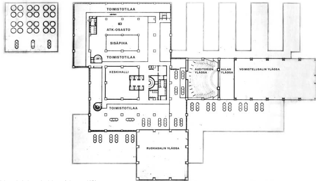
➤ Pohjolan toimitalo, esittelykuva, 2. kerros, 1970 Arkkitehtuuritoimisto Heikki Castrén & Co. AmA
