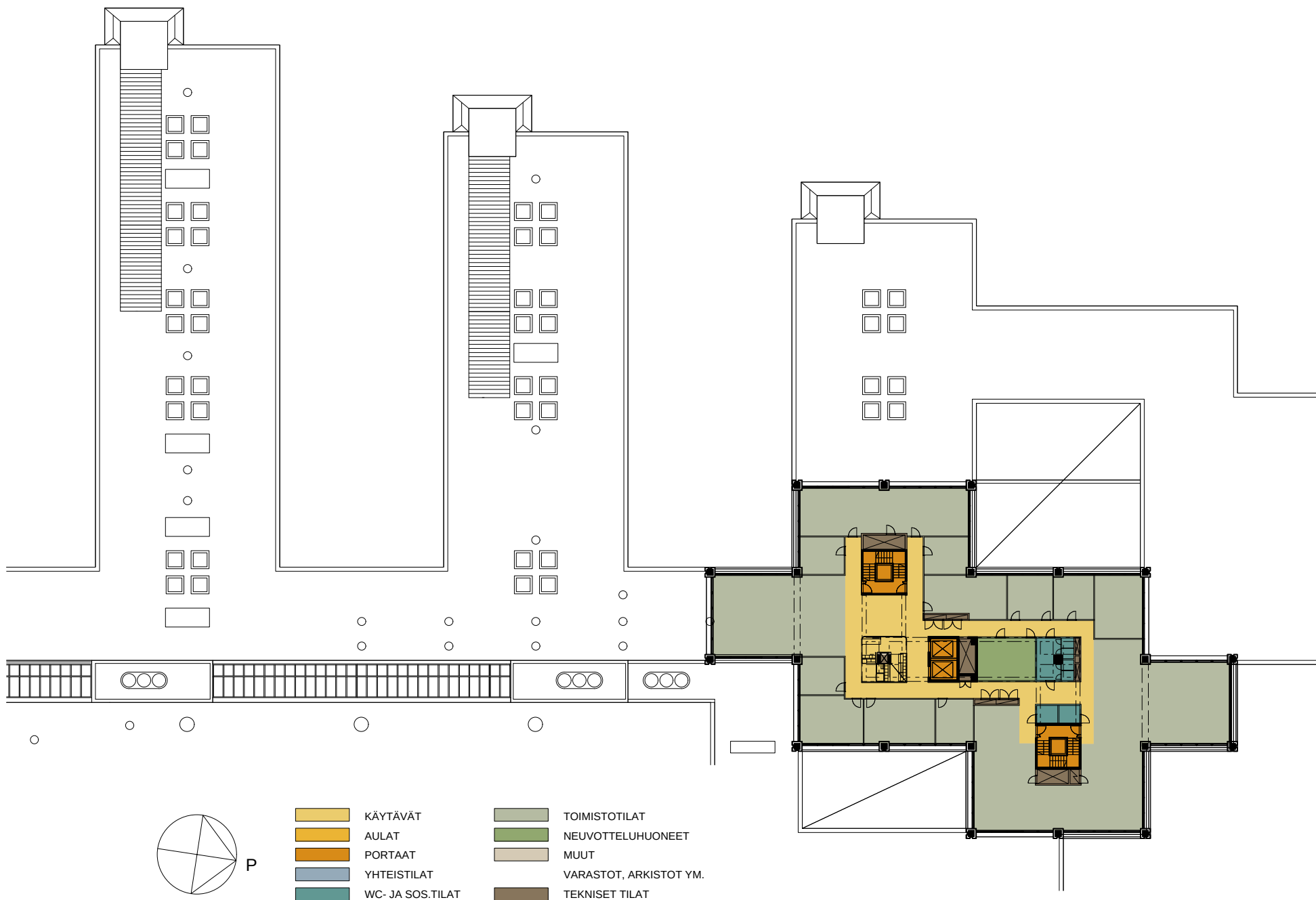
4. KRS – LAAJENNUS, 1/500
